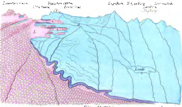
Fig. 2. Keilförmiges gegenseitiges Ineinandereingreifen von Gneiss und Kalk am Gstellhorn.
